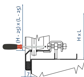
Fixováno skrytým držákem
