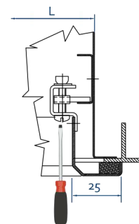
Upevnění skrytým držákem na univerzální přípojevací box.
