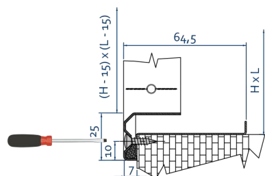
Fixováno viditelným šroubem
