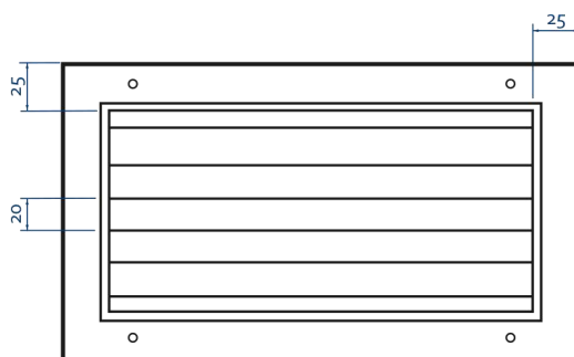
1. Rozměry ventilačních mříží typu CN a CNK
