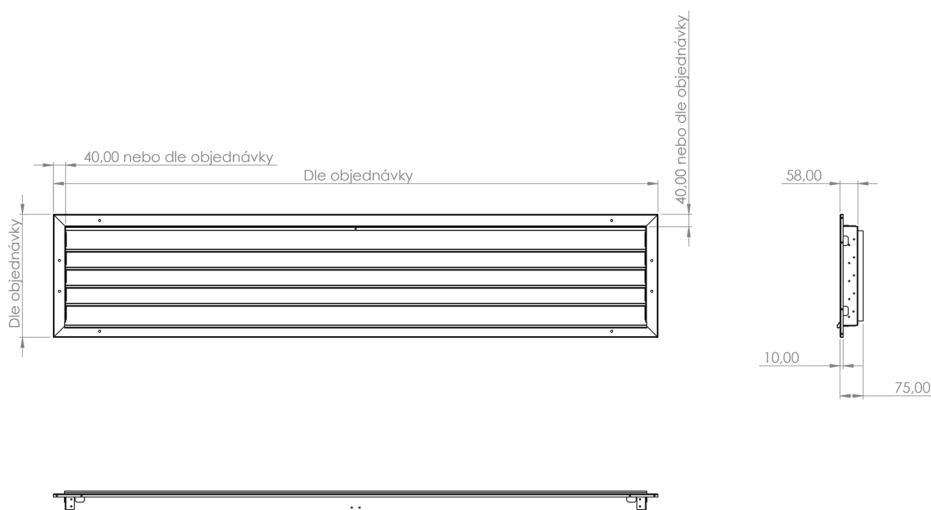
1. Rozměry protidešťové žaluzie
