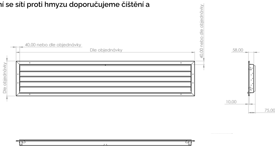
1. Rozměry protidešťové žaluzie
