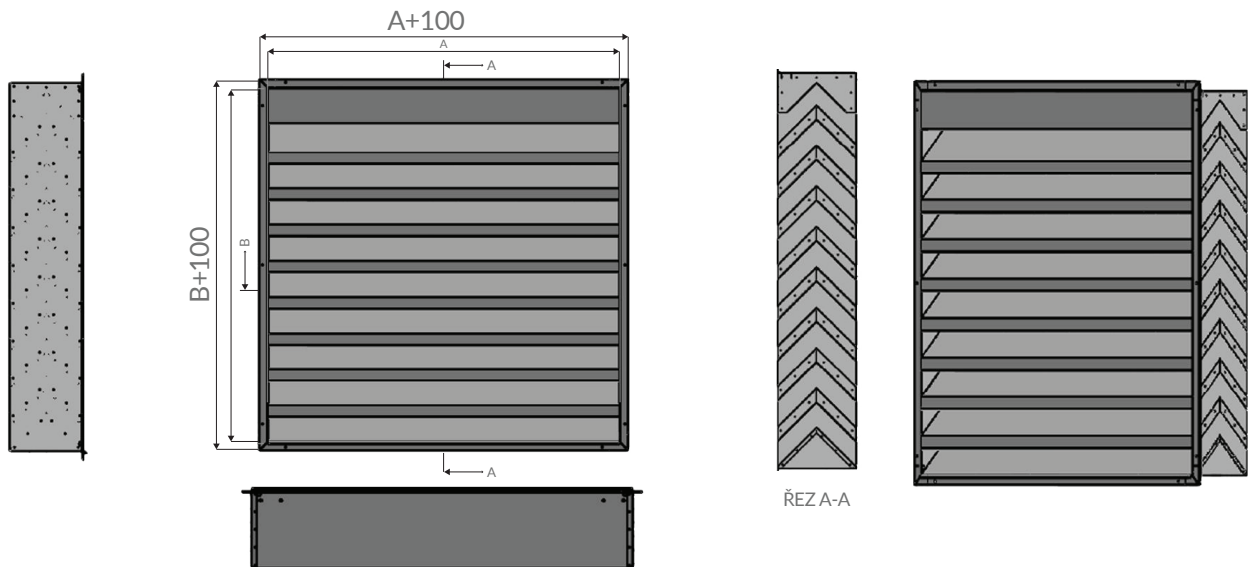
Příklad PHZ na zakázku bez čelního rámu
